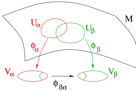
Figure 1: Übergangsabbildungen
